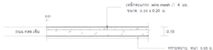
รูปตัด ถนน NOT TO SCALE
