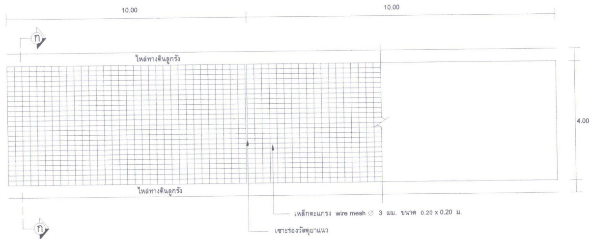
แปลนถนนคอนกรีตเสริมเหล็ก NOT TO SCALE
